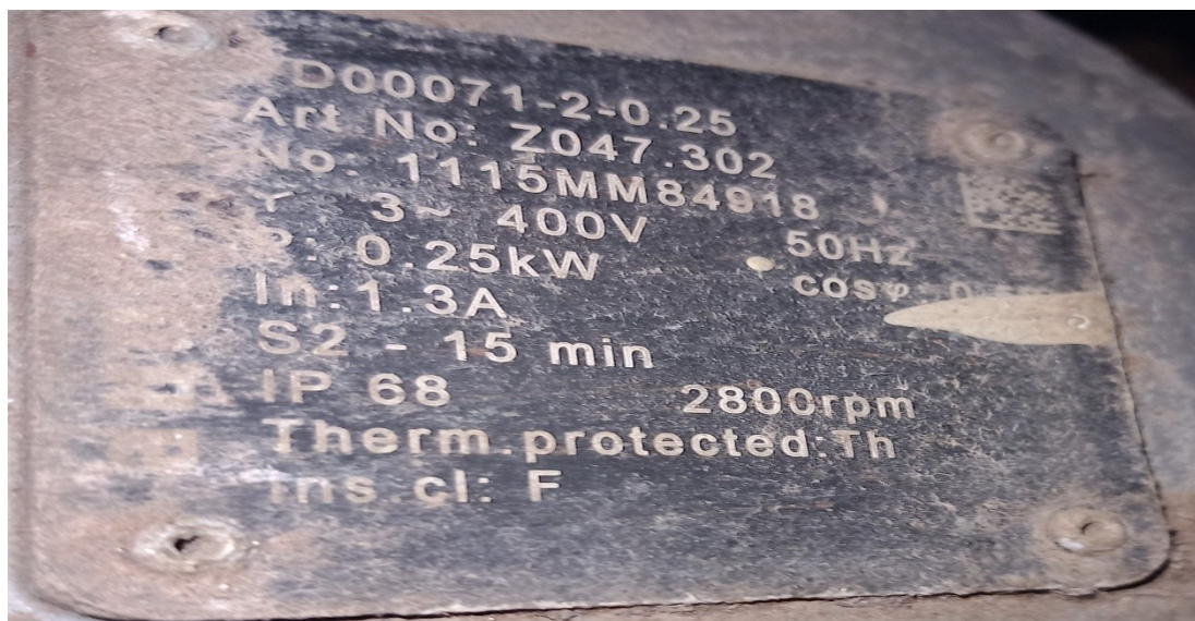
VD00071-2-0.25 motor
