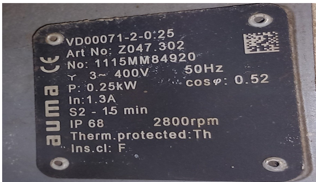
VD00071-2-0.25 motor
