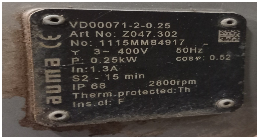
VD00071-2-0.25 motor
