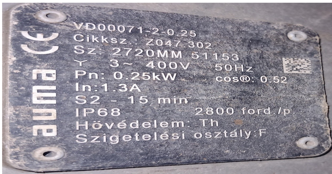
VD00071-2-0.25 motor
