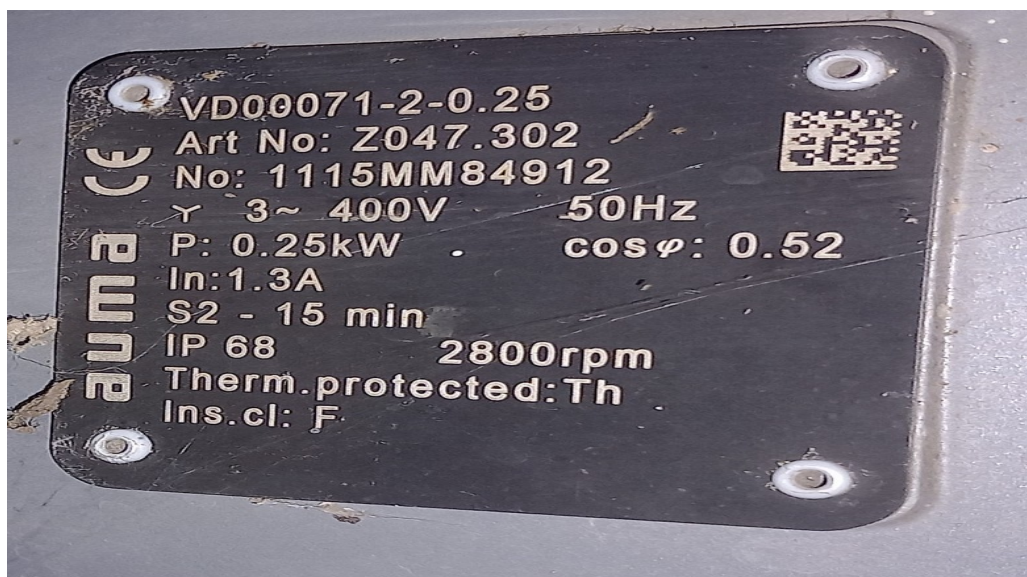
VD00071-2-0.25 motor
