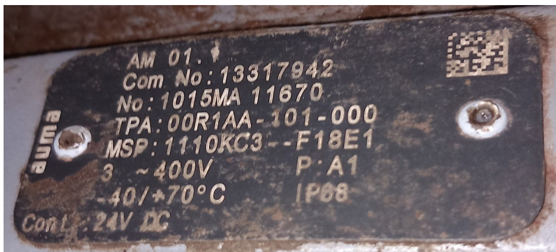
AM 01.1 vezérlő
