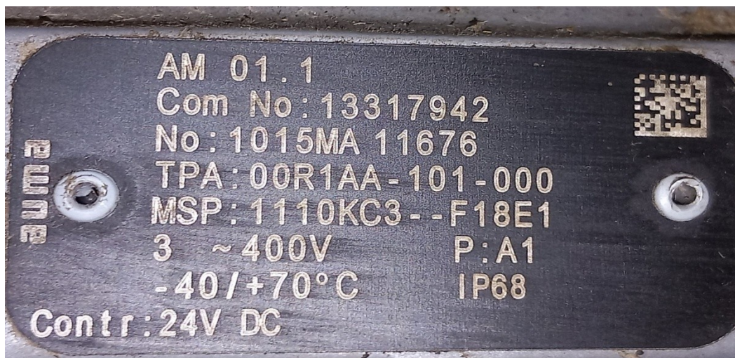
AM 01.1 vezérlő
