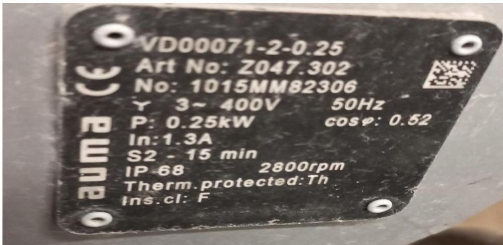
VD00071-2-0.25 motor
