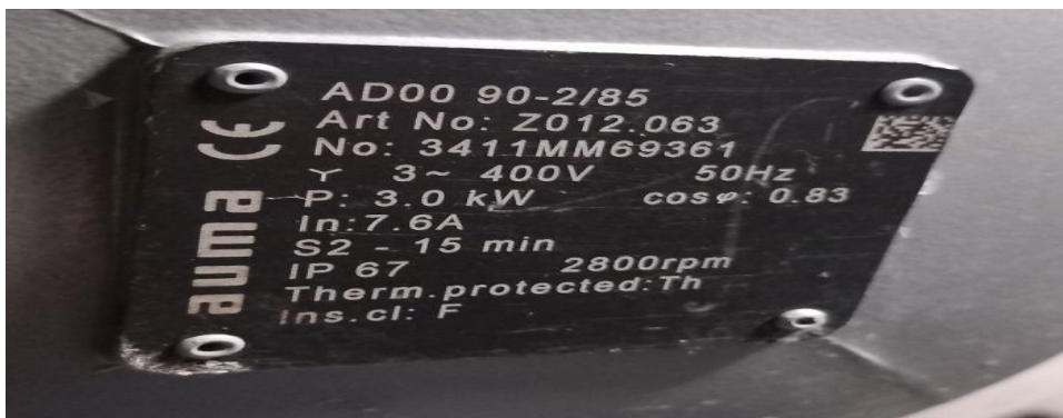
AD00 90-2/85 motor
