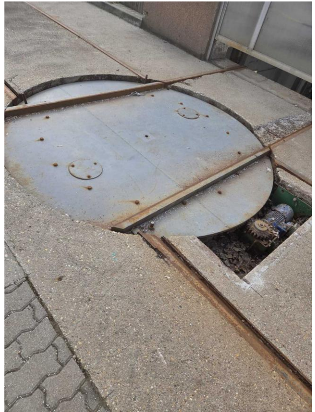
2-es emelőasztal motoros konténerforgató korong korong.
